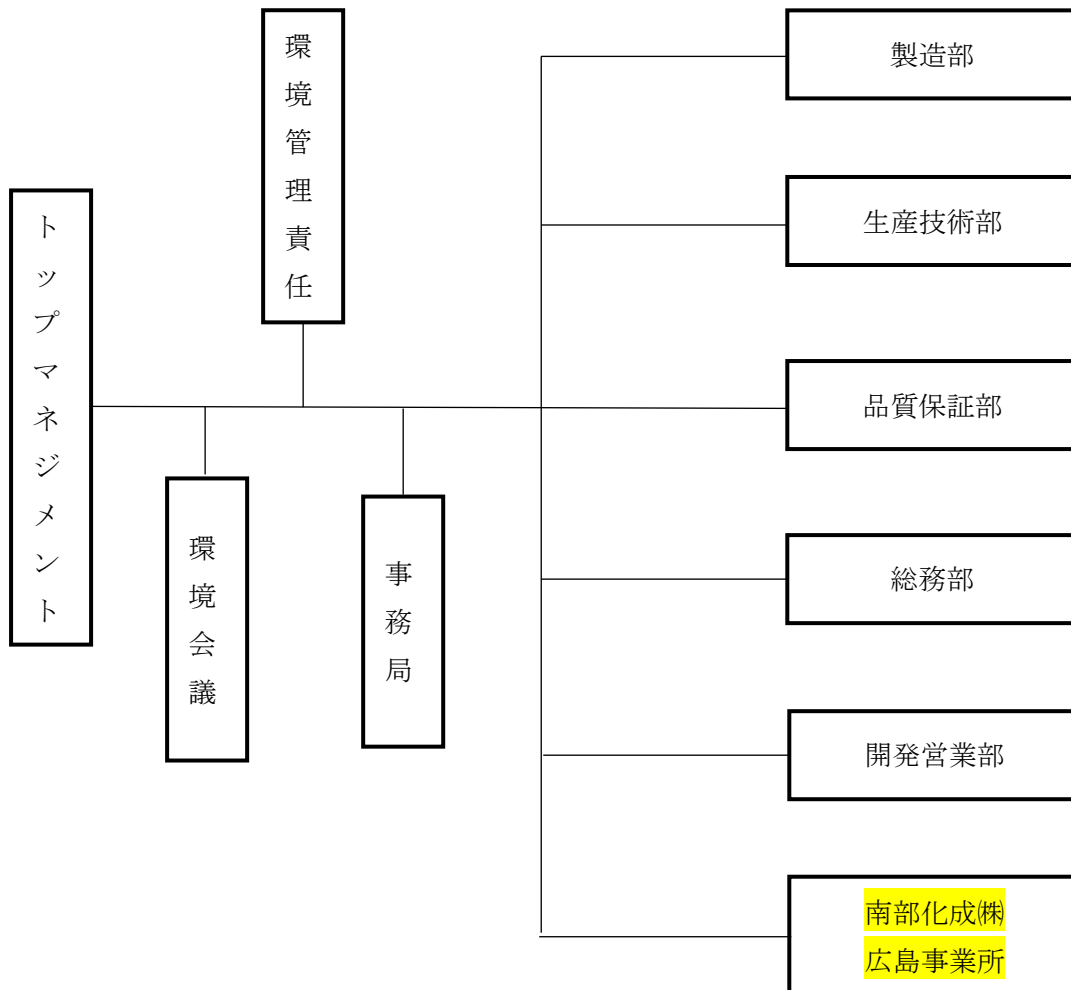
図 1 : 組織図
